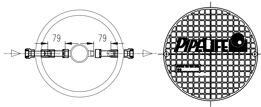
Фиксиран капак DN400, EN124, A15
